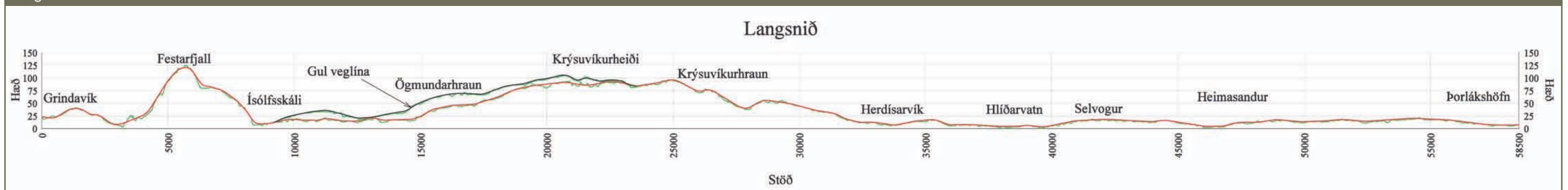
Mynd 24. Langsnið milli Grindavíkur og Þorlákshafnar - Rauð og gul veglína
